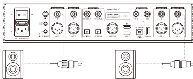
RCA连接功放或者有源音箱示意图
