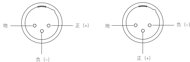
设置正向时端口极性示意
