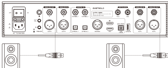
XLR连接功放或者有源音箱示意图
